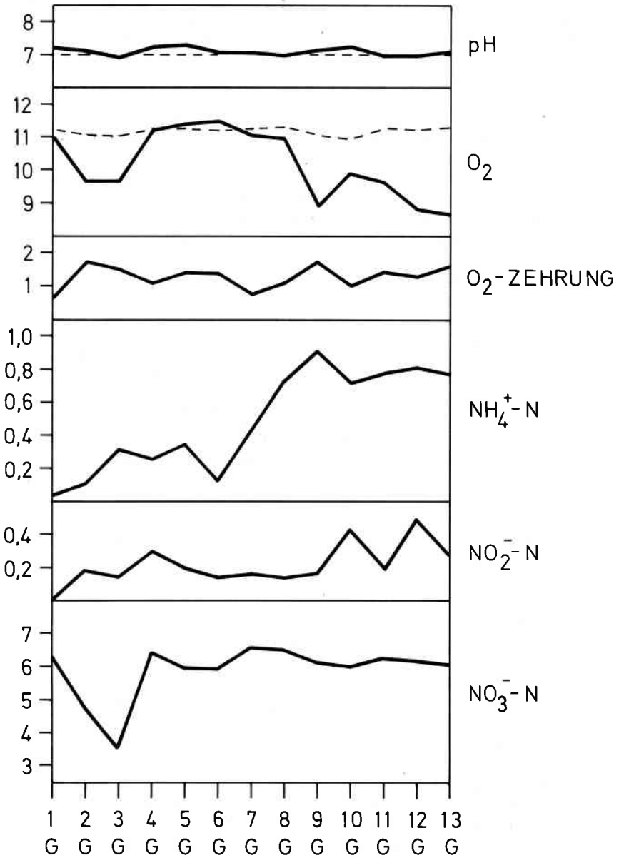
Abb. 4: Physikalisch-chemische Kenndaten des Gewinghauserbaches. Für die Probestellen 1-13 sind die jeweiligen Mittelwerte aus 12 Messungen des Untersuchungszeitraumes April 1977 - Februar 1978 dargestellt. Konzentrationsangaben in mg/l.
