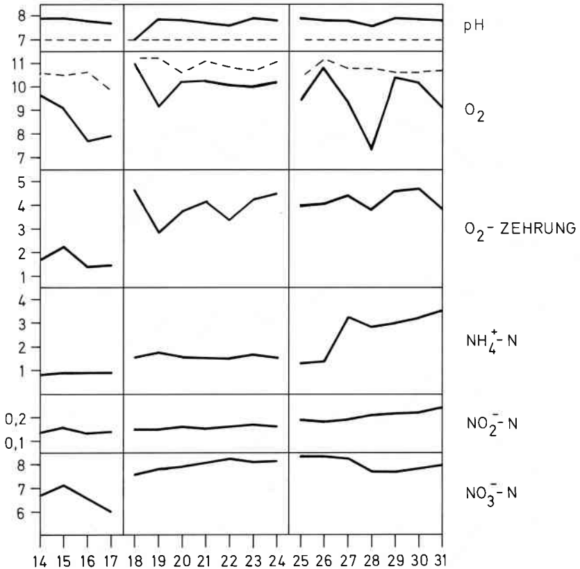
Abb. 3: Physikalisch-chemische Kenndaten der Elbe. Für die Probestellen 14–17 sind die jeweiligen Mittelwerte aus 12 Messungen des Untersuchungszeitraumes Juli – Dezember 1975, für die Probestellen 18–31 von Juli 1975 – Juli 1976 dargestellt. Konzentrationsangaben in mg/l.
