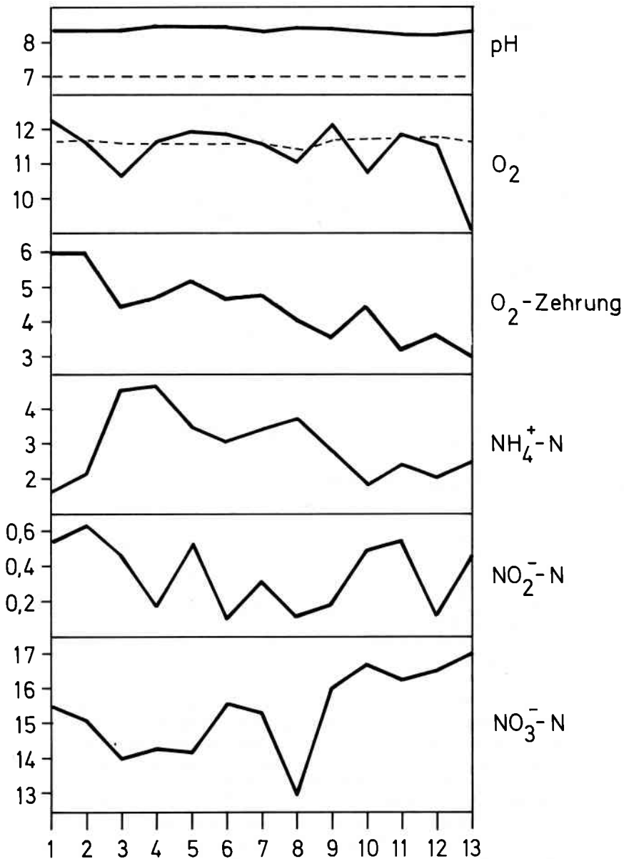
Abb. 2: Physikalisch-chemische Kenndaten der Elbe. Für die Probestellen 1-13 sind die jeweiligen Mittelwerte aus 12 Messungen des Untersuchungszeitraumes September 1976 - März 1977 dargestellt. Konzentrationsangaben in mg/l.
