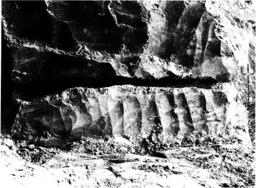
Abb. 3: Das aufgegrabene Höhlenprofil (oben) sowie dessen schematische Darstellung mit Abmessungen (unten). Aufn.: R. SIEBRASSE
