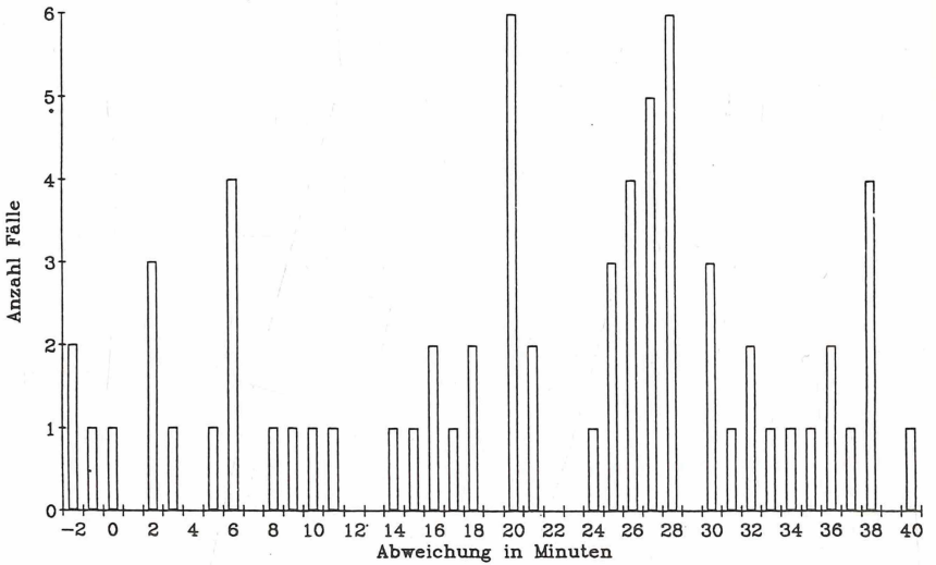
Abb. 9: Abweichung der Erstankunftszeit vom Sonnenaufgang
