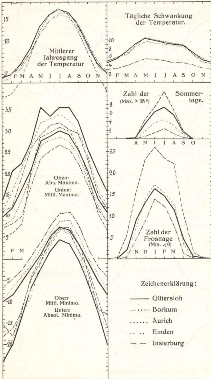
Tafel I. Die Temperaturverhältnisse.
