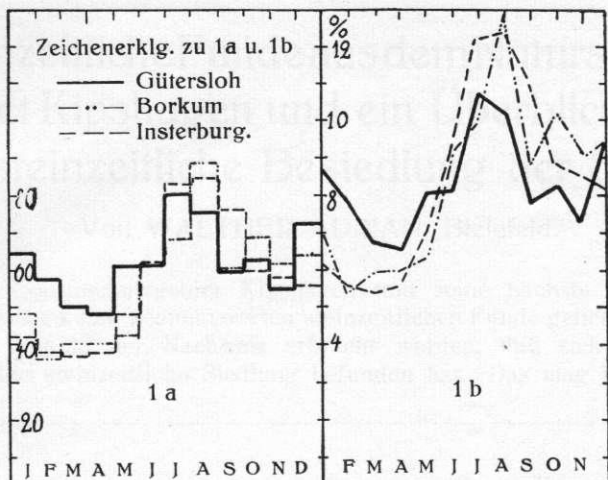
Tafel III. Die Niederschlagsverhältnisse.
