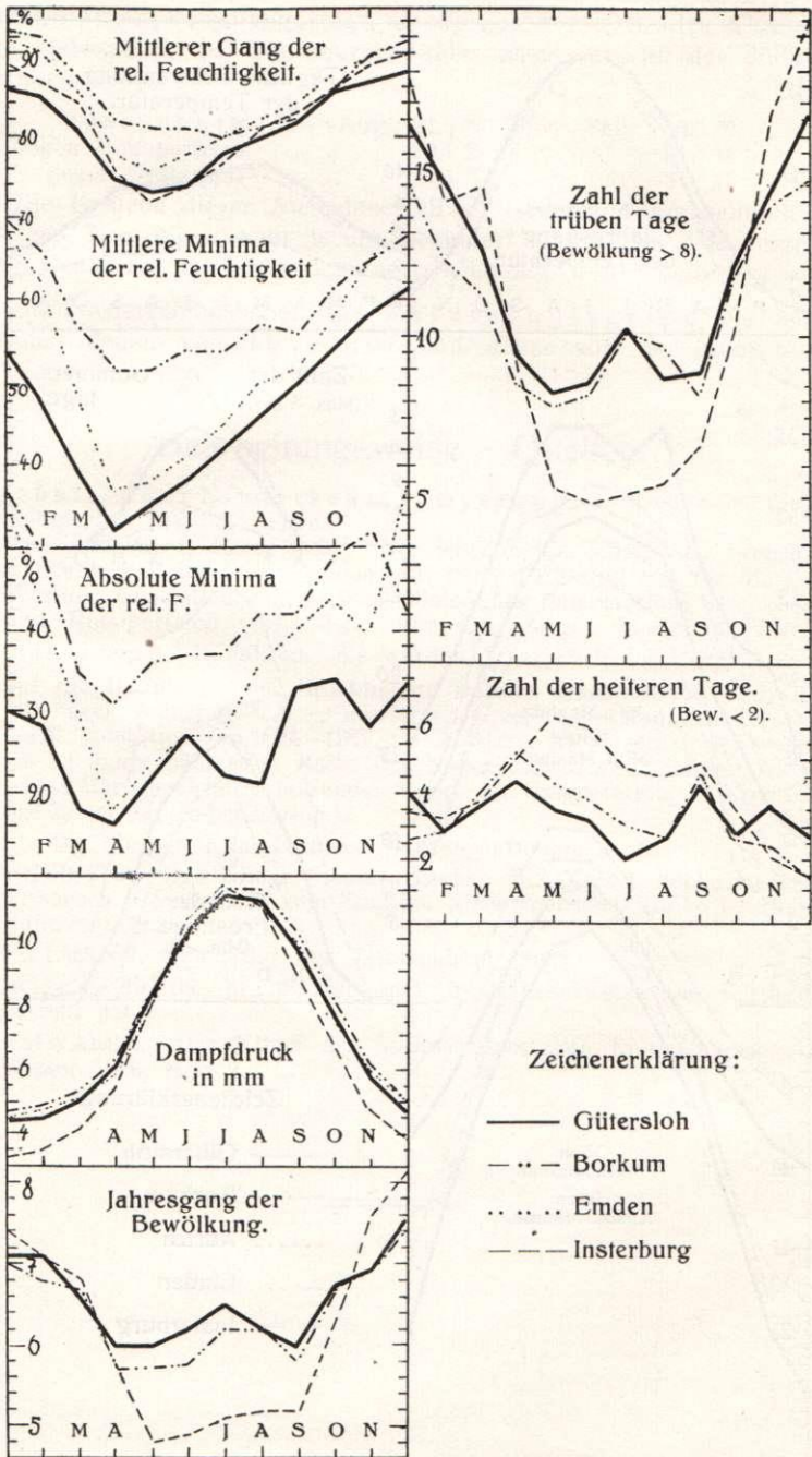
Tafel II. Luftfeuchtigkeit und Bewölkung.
